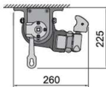
Deckenmontage
